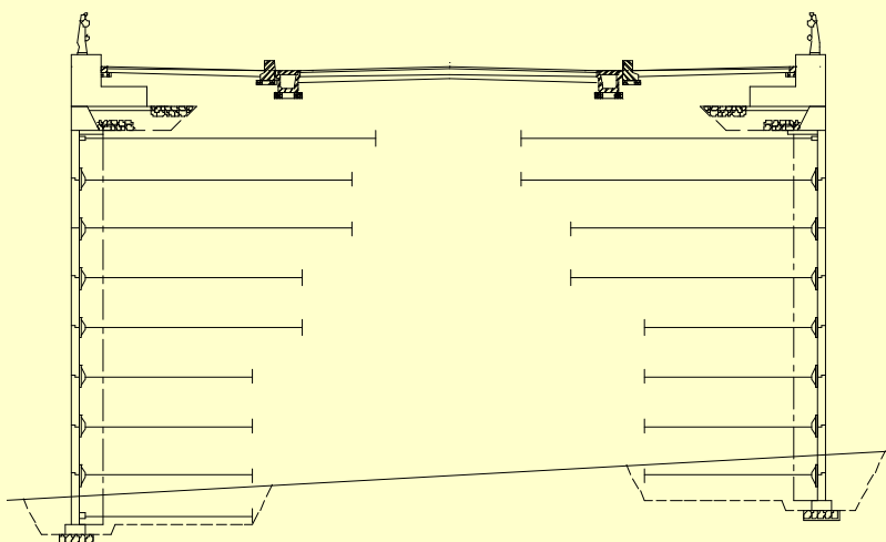
通常タイプ横断図
