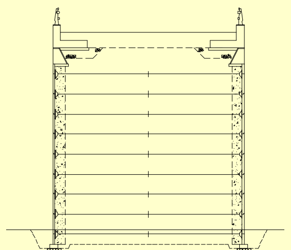
緊結タイプ横断図
