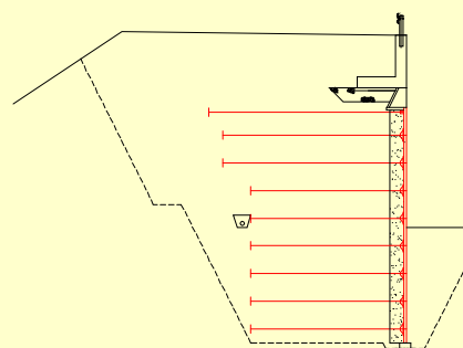
A1橋台右側横断図
