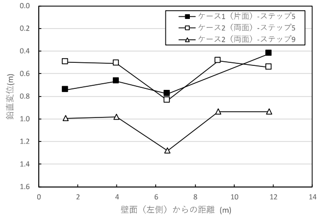
図7 天端の残留鉛直変位（ステップ5及び9）
