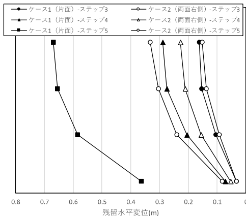
図6 壁面の残留水平変位（ステップ3～5）
